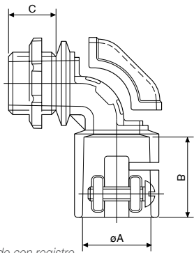
>> Plano Codo con registro
