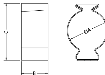
>> Plano Abrazadera tipo Chaveta
