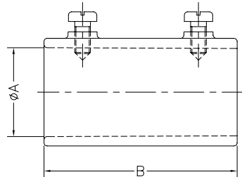
>> Plano Empalme sin rosca
