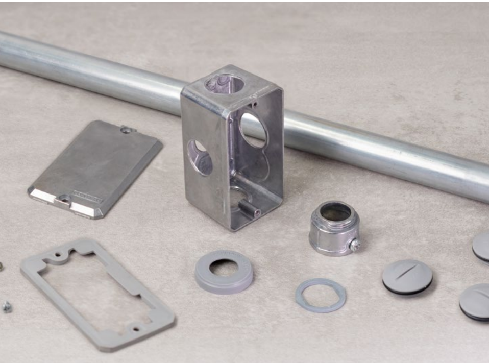
>> Caja Múltiple tipo X y accesorios para grado IP 54.
